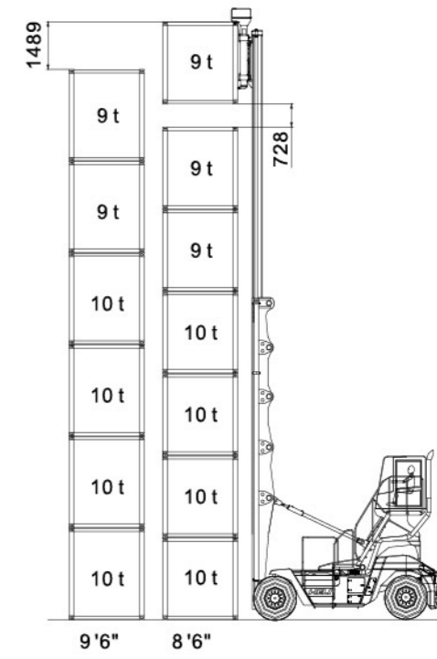
整车负荷图
