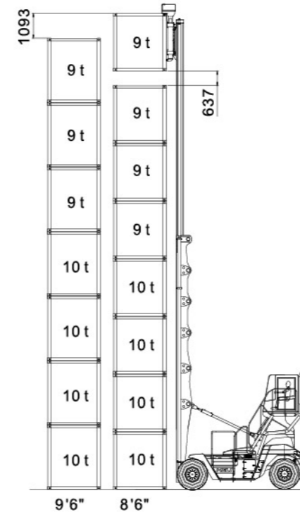
整车负荷图
